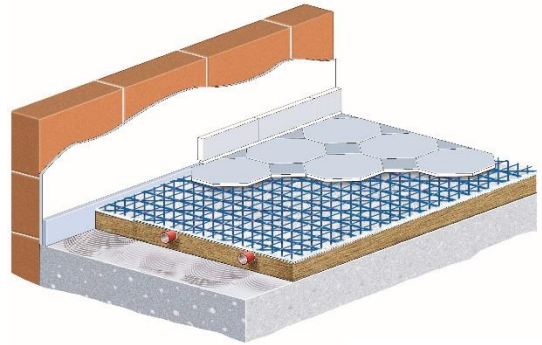
Bild 2 Aufbau Entkopplungsmatte
